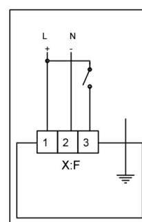
2bodové ovládání
